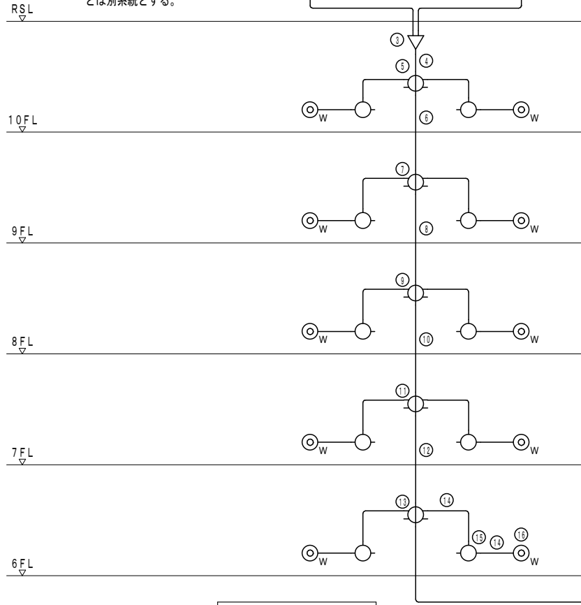
受信システム系統図
