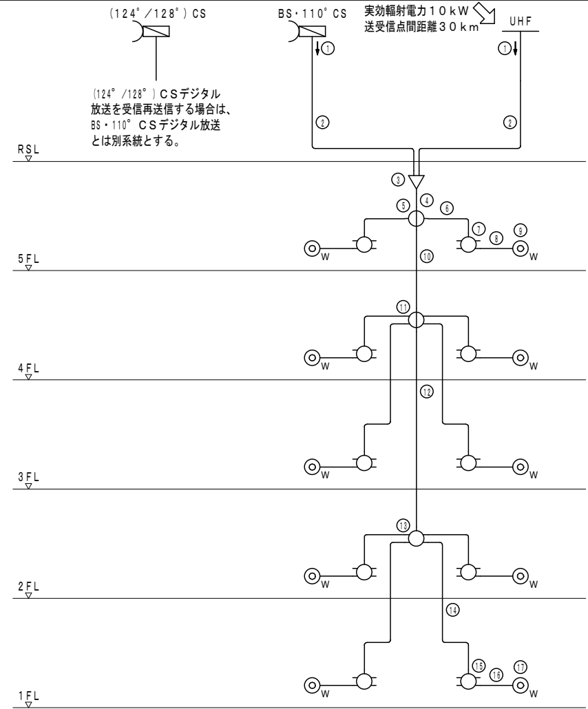
受信システム系統図
