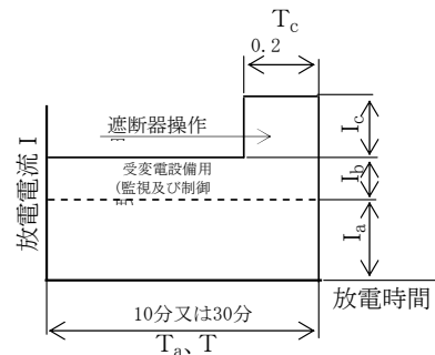
図2-3 蓄電池負荷特性
